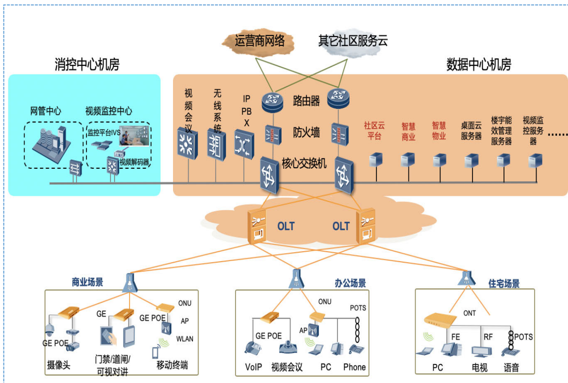
【智能基础设施系统组成图】
